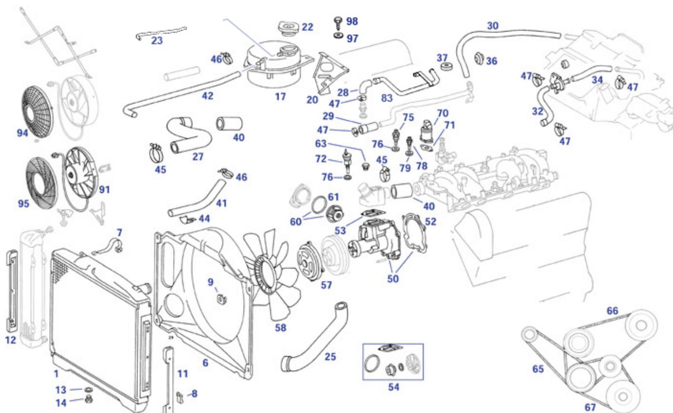
Kühlwasser führende Teile für Eisenguss-V8, hier in Europa-/Standardausstattung: ohne Klimaanlage, ohne Umwälzpumpe.
